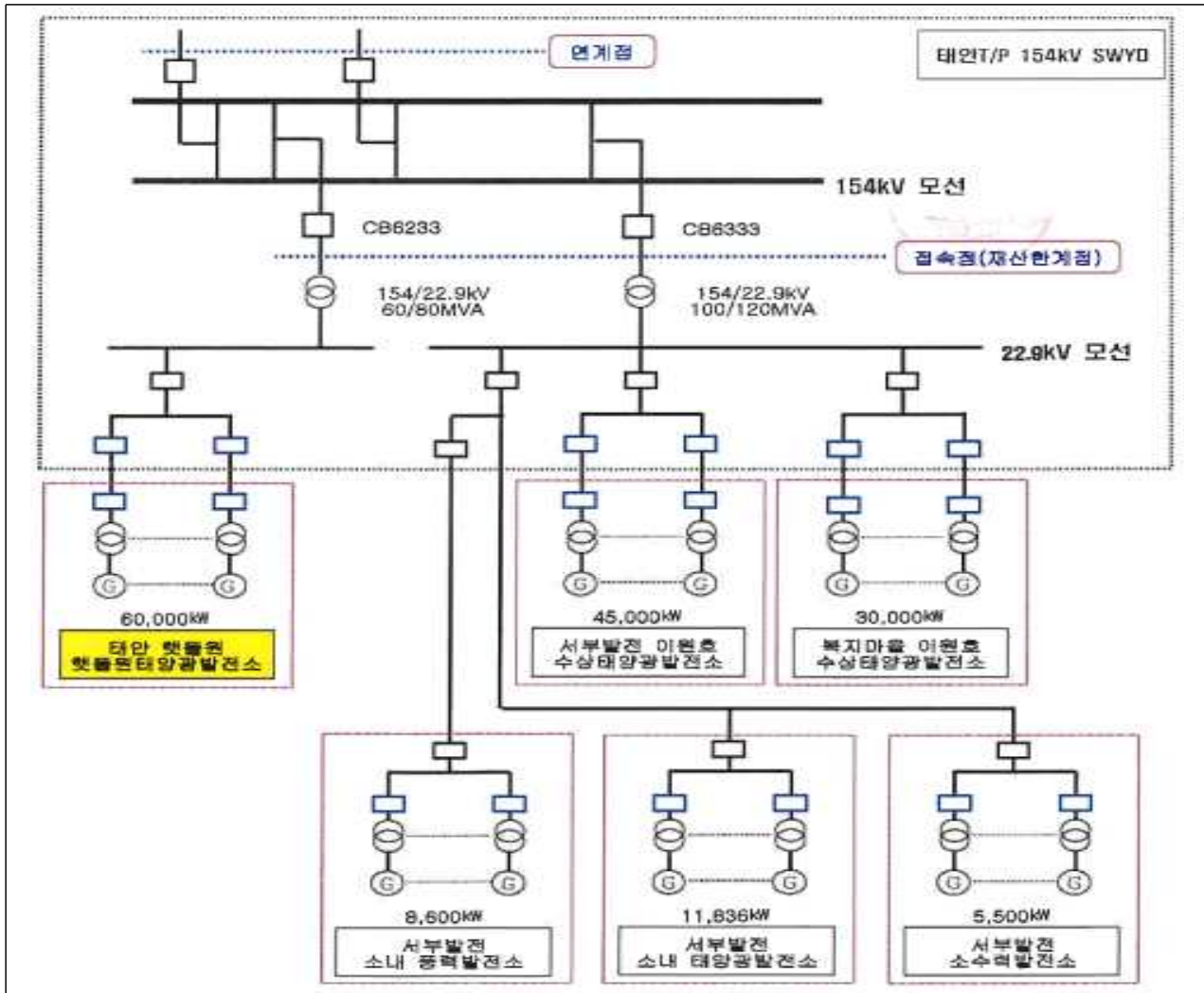
[그림 1] 공동이용 송·변전 전기설비 개요도
